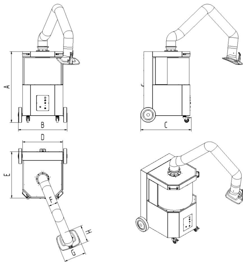
Рис. 7: Габаритный чертеж
