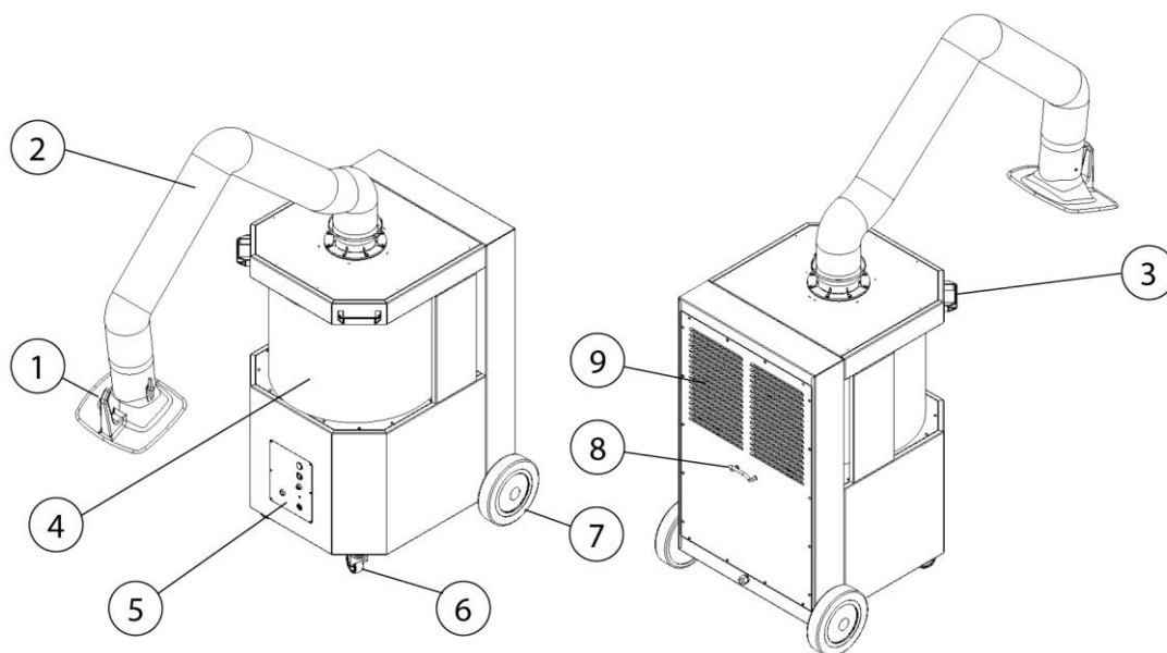
Рис. 1: Позиции на изделии
