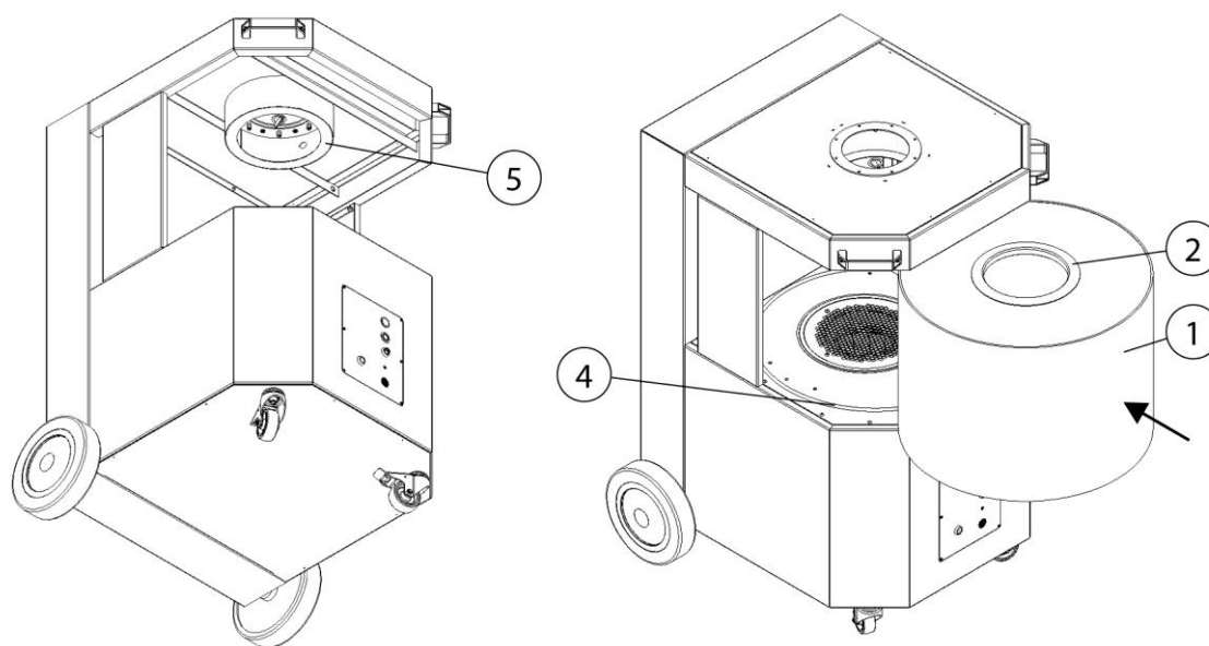
Рис. 6: Замена фильтра - установка фильтрующего элемента
